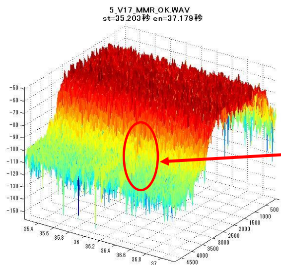
図 6.45 (Outband_IFFT 3次元表示画面)
