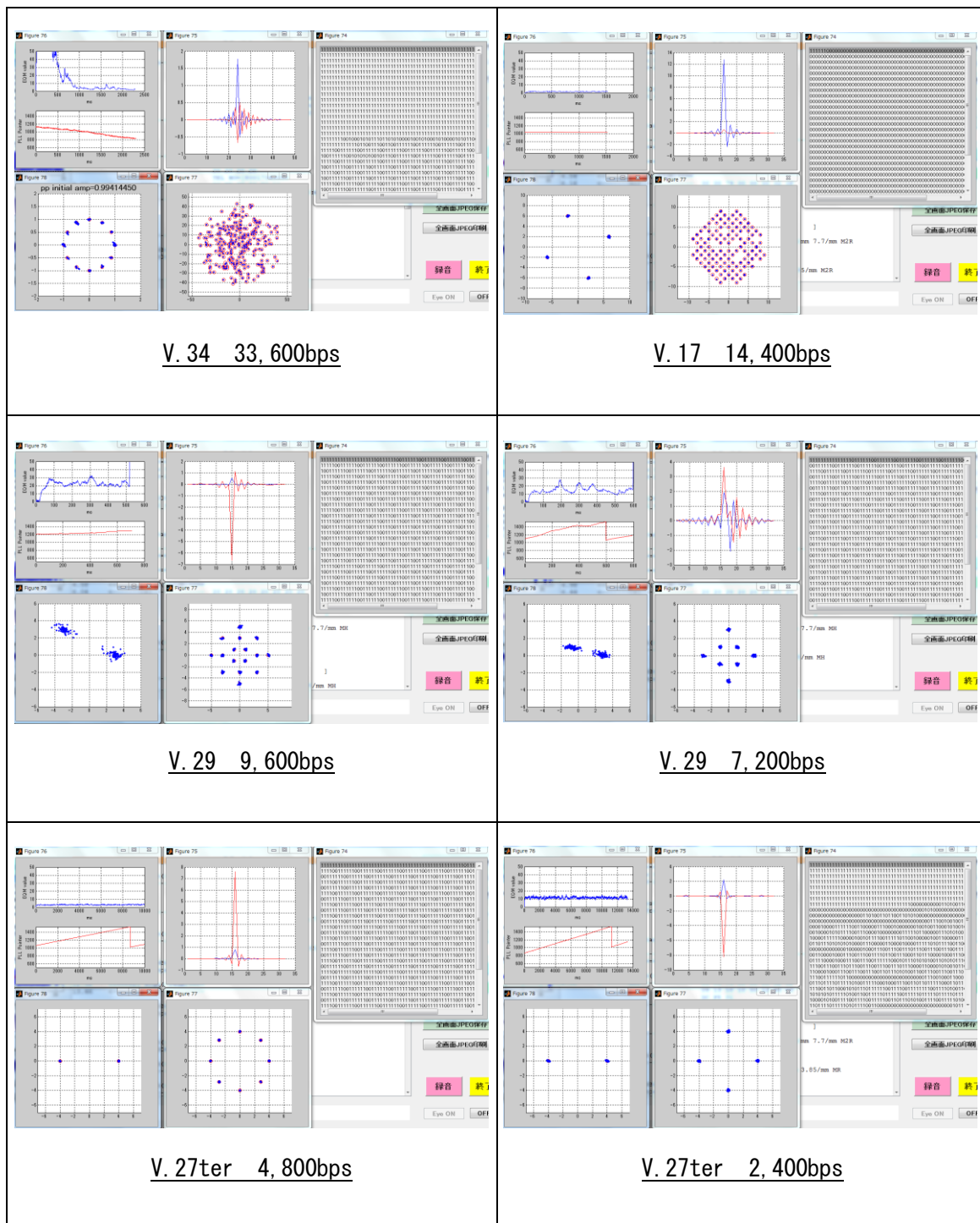
図 6.40 (各通信モードでのアイ・パターン・ジェネレータ)
