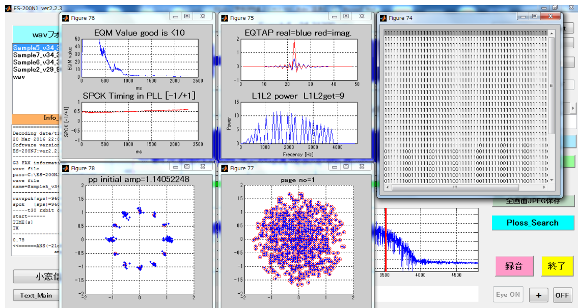
図 6.39 (アイ・パターン・ジェネレータ 画面)
