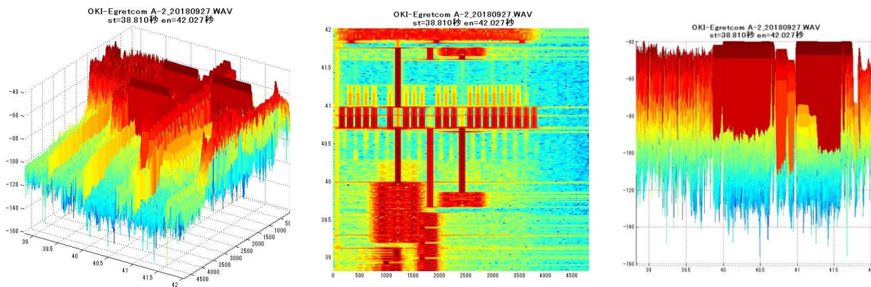
図 6.53 (Outband_IFFT 遠端エコー観測 3次元表示)
