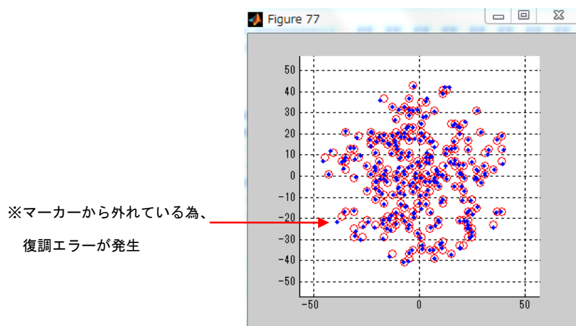
図 6. 41 (復調エラー発生時の Constellation)
