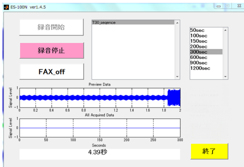
図 6. 29 (録音中画面)
