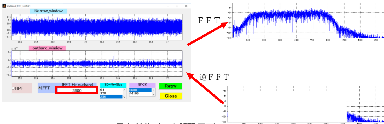
図 6. 44 (Outband_IFFT 画面)
