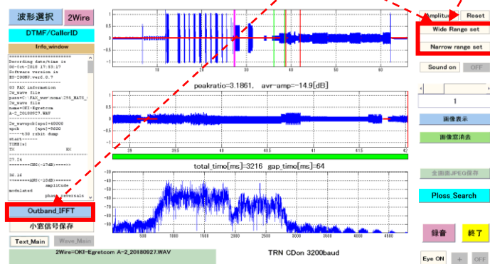
図 6.52 (Outband_IFFT 遠端エコー観測)
