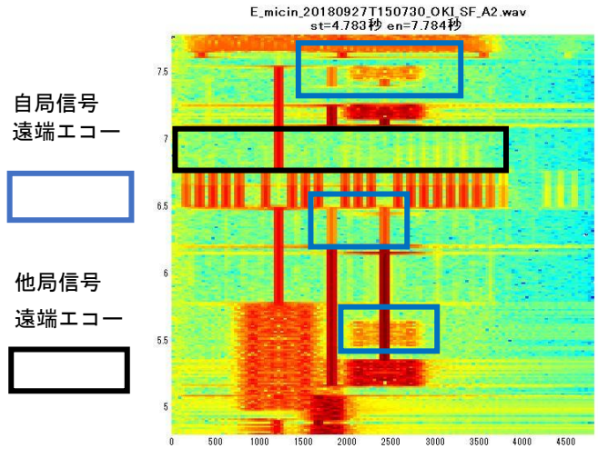
受信FAX-録音 (v34) -XY表示
